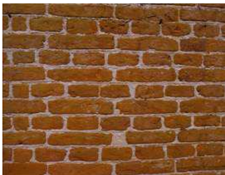
Caramizi pline Rost orizontal si vertical de mortar
